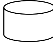
database
